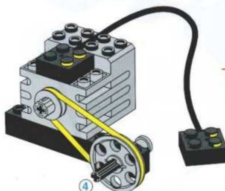
Using pulley wheels Rollenräder verwenden
