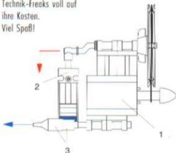
Abb. 3a: Ausblasen
