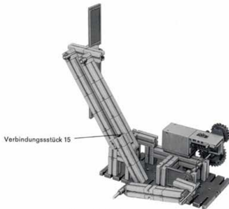
37.2 Rückansicht
