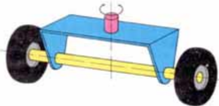
Drehschemel-Lenkung
