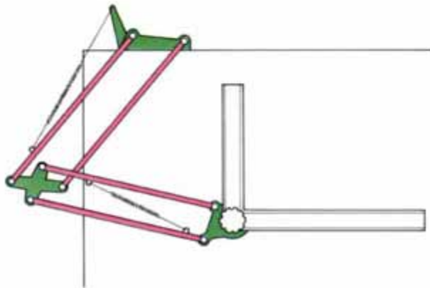
Zeichenmaschine
