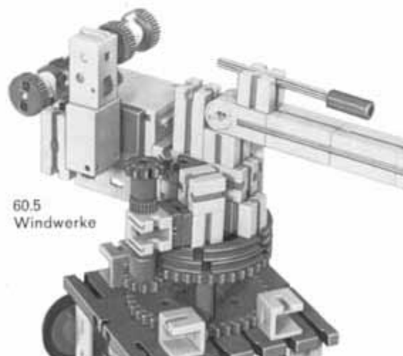
60.5 Teilansicht
