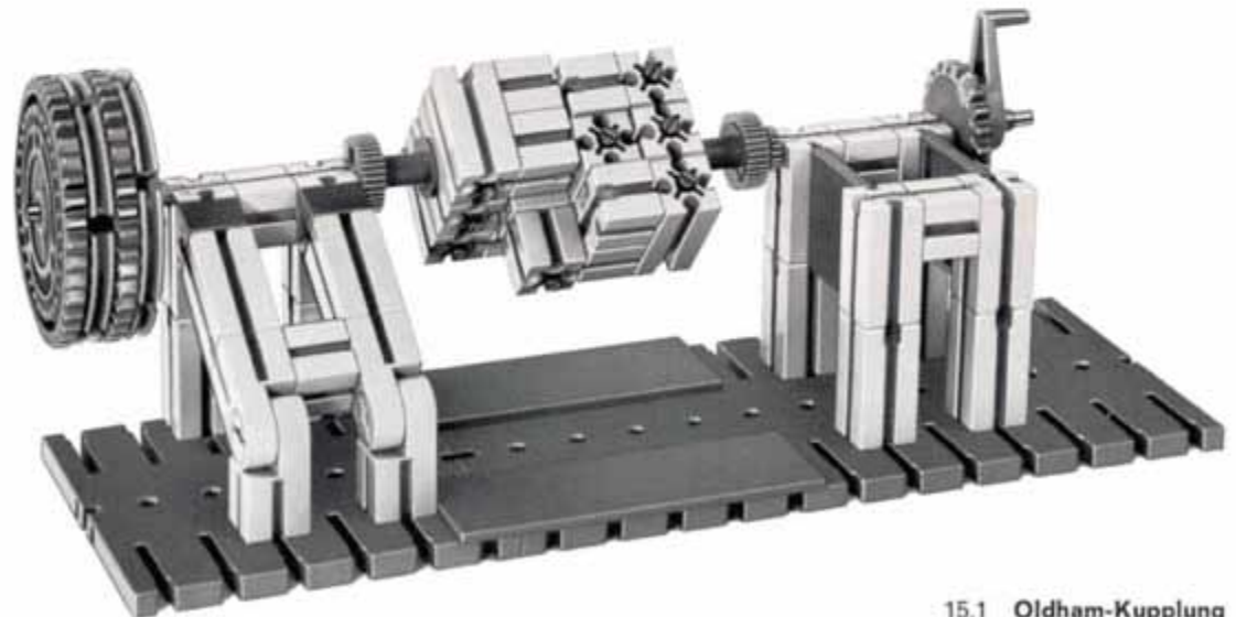
15.1 Oldham-Kupplung
