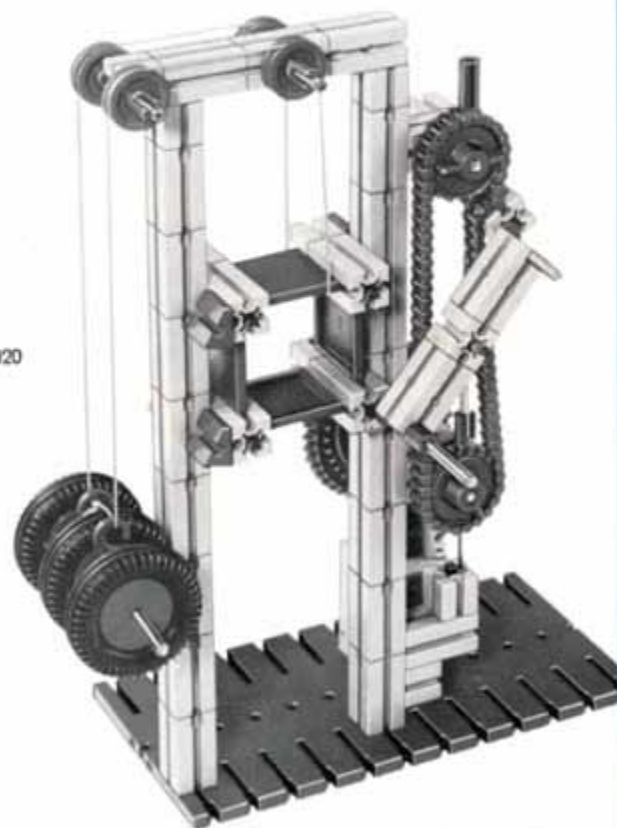
43.1 Aufzug
