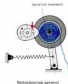
46.2 Reibradantrieb getrennt
