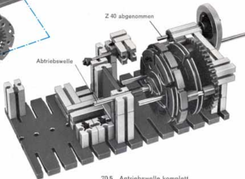
70.5 Antriebswelle komplett
