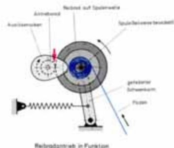
46.1 Reibradantrieb in Funktion
