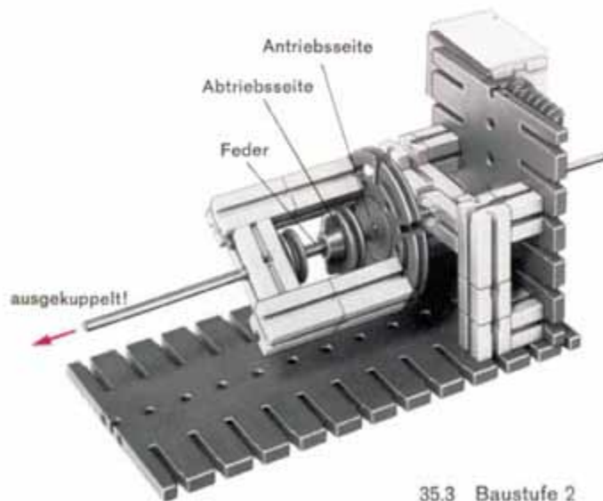
35.3 Baustufe 2
