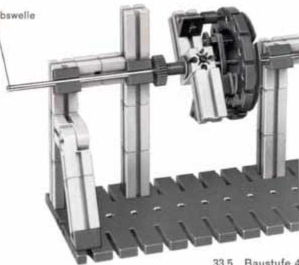
33.5 Baustufe 4
