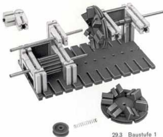
29.3 Baustufe 1
