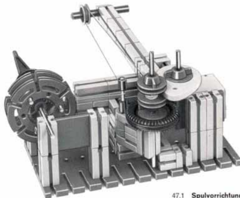
47.1 Spulvorrichtung
