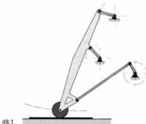
Prinzip der Glanzstoßmaschine
