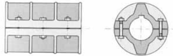
5.1 Schalenkupplung
