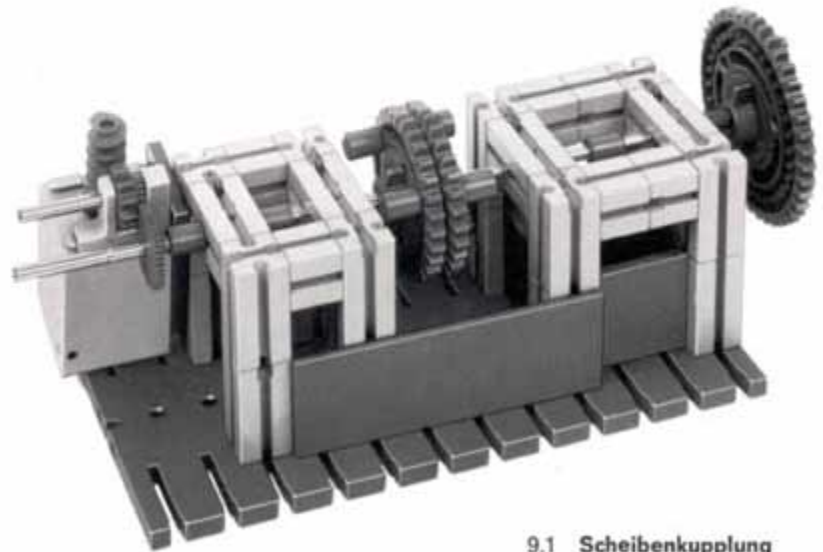
9.1 Scheibenkupplung
