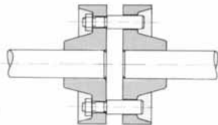
10.2 Bolzenkupplung
