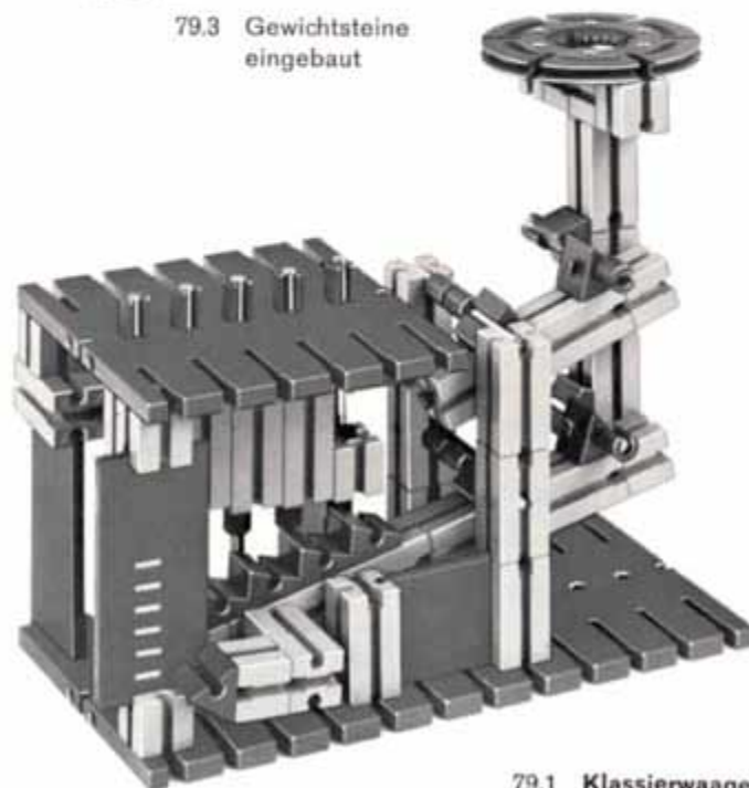
79.1 Klassierwaage
