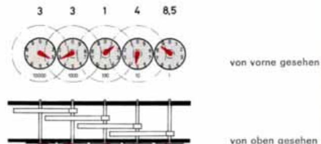
58.1 Analoganzeige
