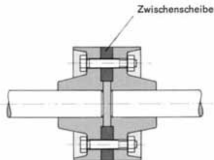
8.2 Scheibenkupplungen
