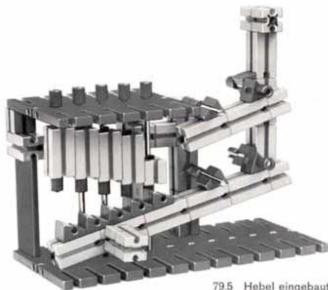
79.5 Hebel eingebaut
