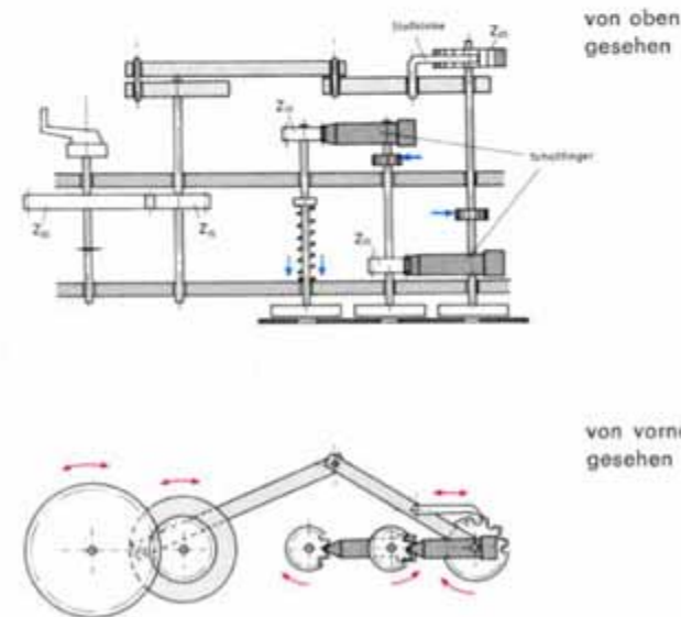
64.1 Zählwerk 0–999, addierend
