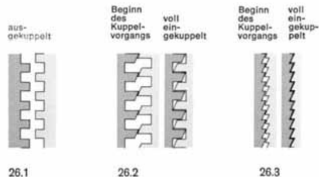
Klauenkupplungen
