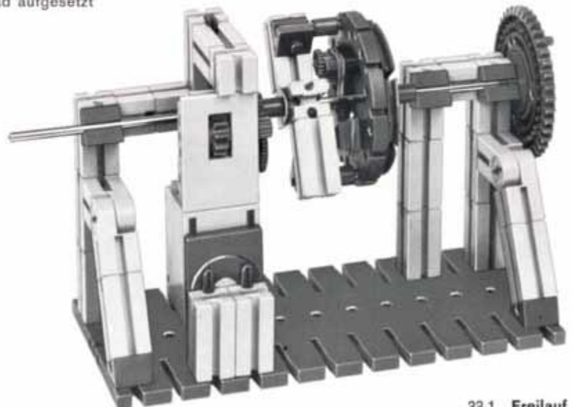
33.1 Freilauf
