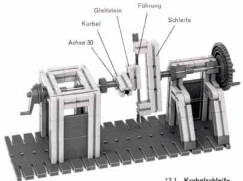
13.1 Kurbelschleife
