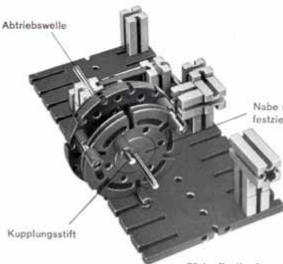
70.4 Freilauf montiert
