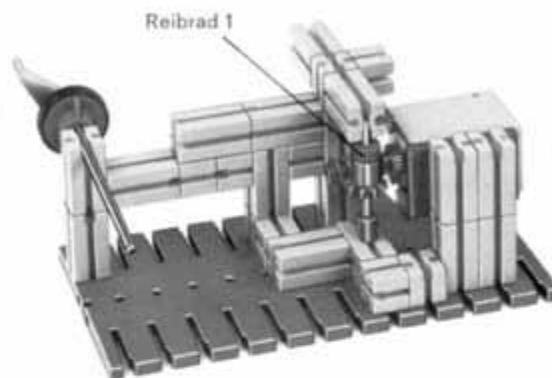
47.2 Baustufe 1
