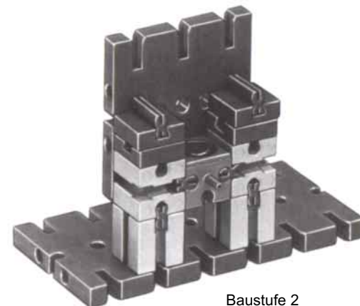
Baustufe 2
