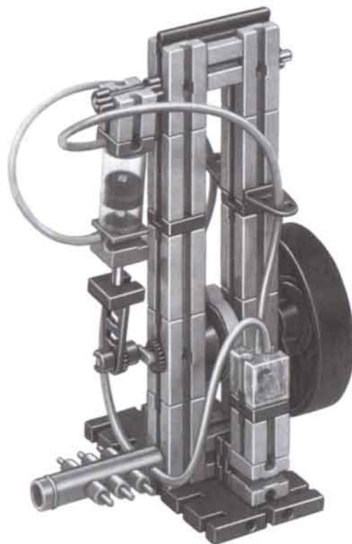
Rückansicht
