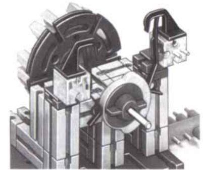
Detail: Ventilsteuerung
