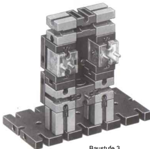
Baustufe 3
