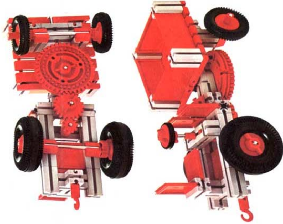
Fahrzeug mit Knicklenkung vehicle with articulated steering chariot à direction articulée veicolo a guida articolata voertuig met knikbesturing
